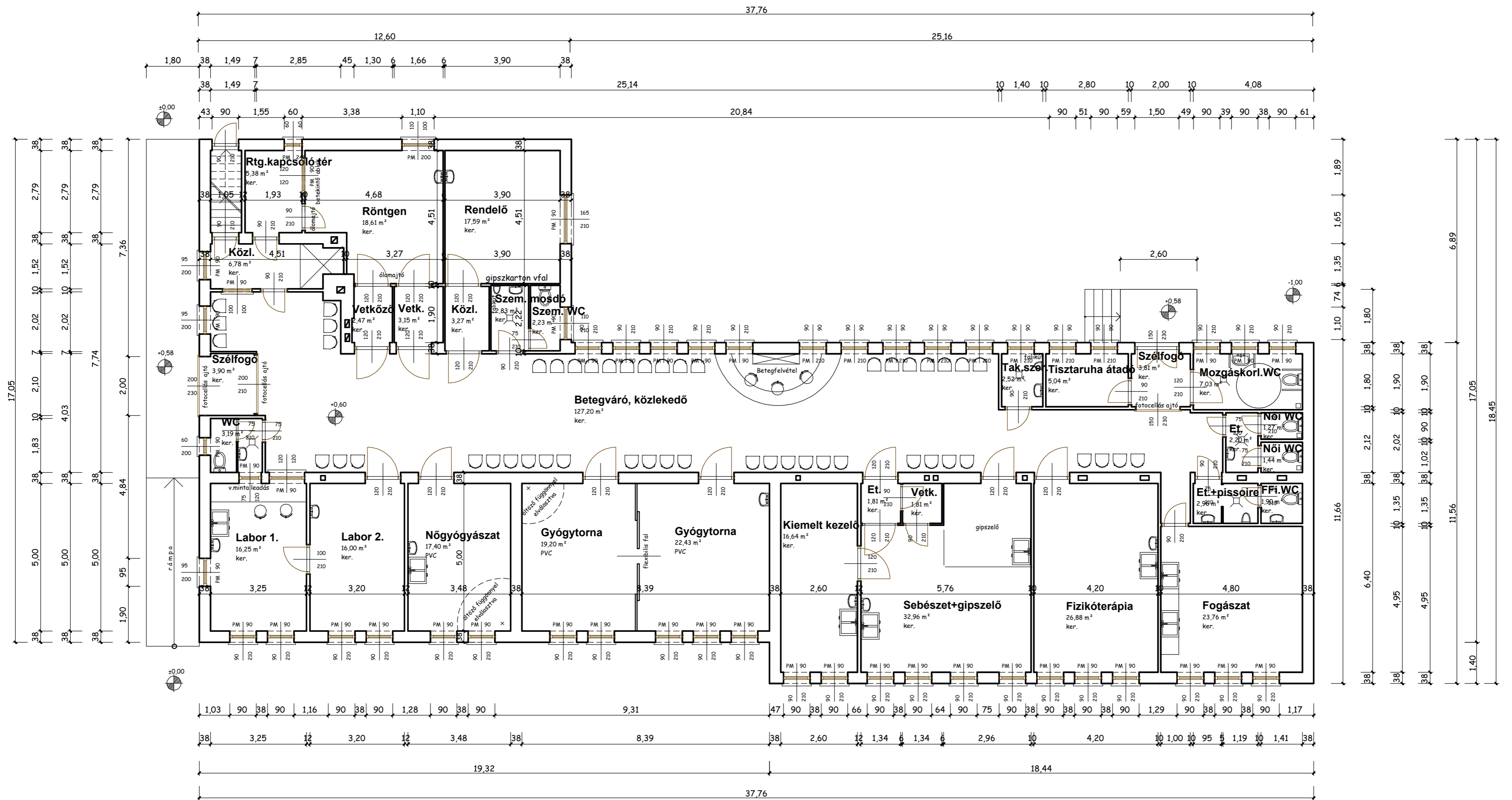
Tervezett fszt-i alaprajz 'A' épület
